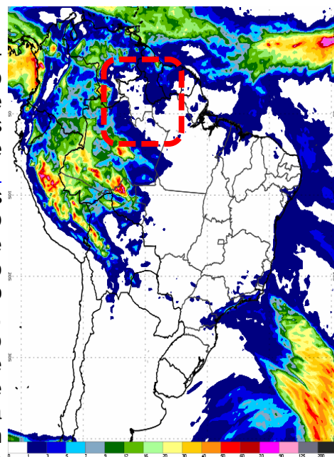
Figura 3 – Modelo de precipitação COSMO (7 x 7km): https://vime.inmet.gov.br/CO
