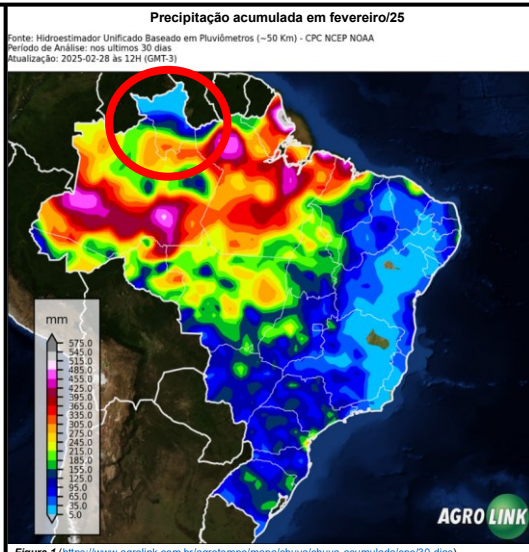
Figura 1 ( https://www.agrolink.com.br/agrotempo/mapa/chuva/chuva-acumulada/cpc/30-dias )
