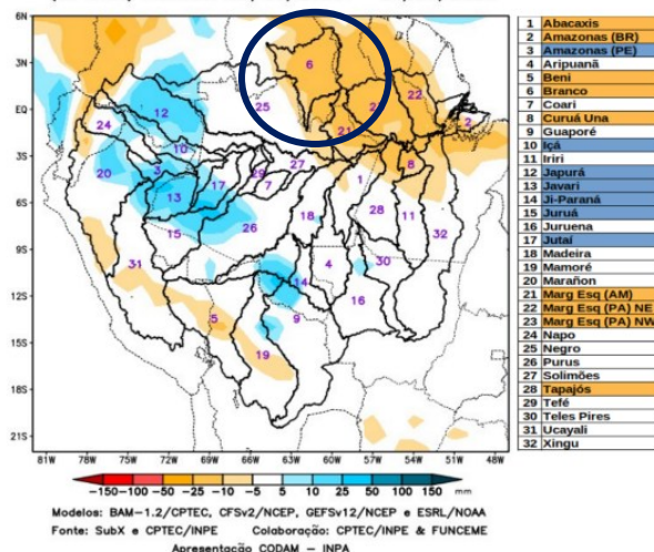
PREVISÃO SUBSAZONAL-MULTIMODELO CALIBRADO Anomalia (mm) de Precipitação Acumulada (07 Dias) Período: 02/09/2026 – 08/09/2026
