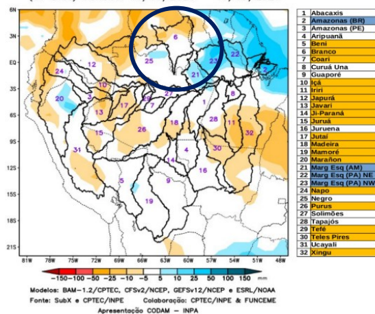
PREVISÃO SUBSAZONAL—MULTIMODELO CALIBRADO Anomalia (mm) de Precipitação Acumulada (07 Dias) Período: 13/05/2026 – 19/05/2026
