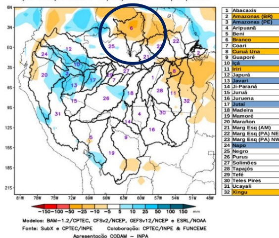
PREVISÃO SUBSAZONAL – MULTIMODELO CALIBRADO Anomalia (mm) de Precipitação Acumulada (07 Dias) Período: 13/05/2026 – 19/05/2026
