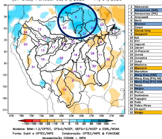
PREVISÃO SUBSAZONAL—MULTIMODELO CALIBRADO Anomalia (mm) de Precipitação Acumulada (07 Dias) Período: 08/04/2026 - 14/04/2026
