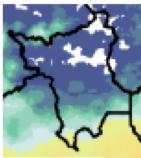
Figura 1 ( https://clima1.cptec.inpe.br/monitoramento/brasil/pt )
