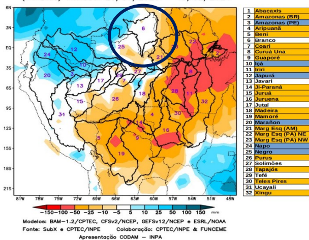
PREVISÃO SUBSAZONAL—MULTIMODELO CALIBRADO Anomalia (mm) de Precipitação Acumulada (14 Dias) Período: 28/01/2026 – 10/02/2026
