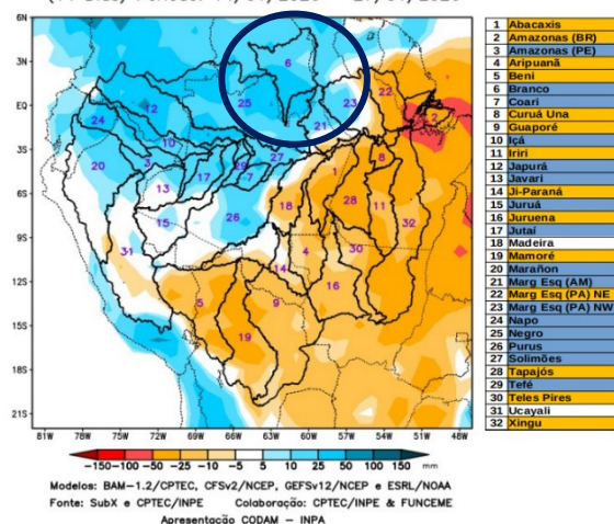
PREVISÃO SUBSAZONAL—MULTIMODELO CALIBRADO Anomalia (mm) de Precipitação Acumulada (14 Dias) Período: 14/01/2026 – 27/01/2026
