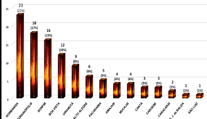
Focos de fogo por município em novembro/25 Total: 107 Focos (0,7% do total Brasil: 16277 focos = 16ª posição)
