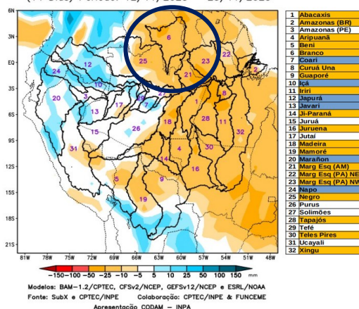
PREVISÃO SUBSAZONAL—MULTIMODELO CALIBRADO Anomalia (mm) de Precipitação Acumulada (14 Dias) Período: 12/11/2025 – 25/11/2025
