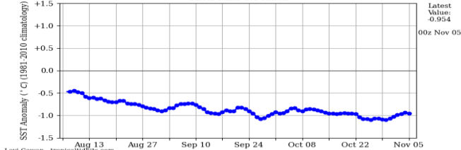
CDAS Niño 3.4 Index
