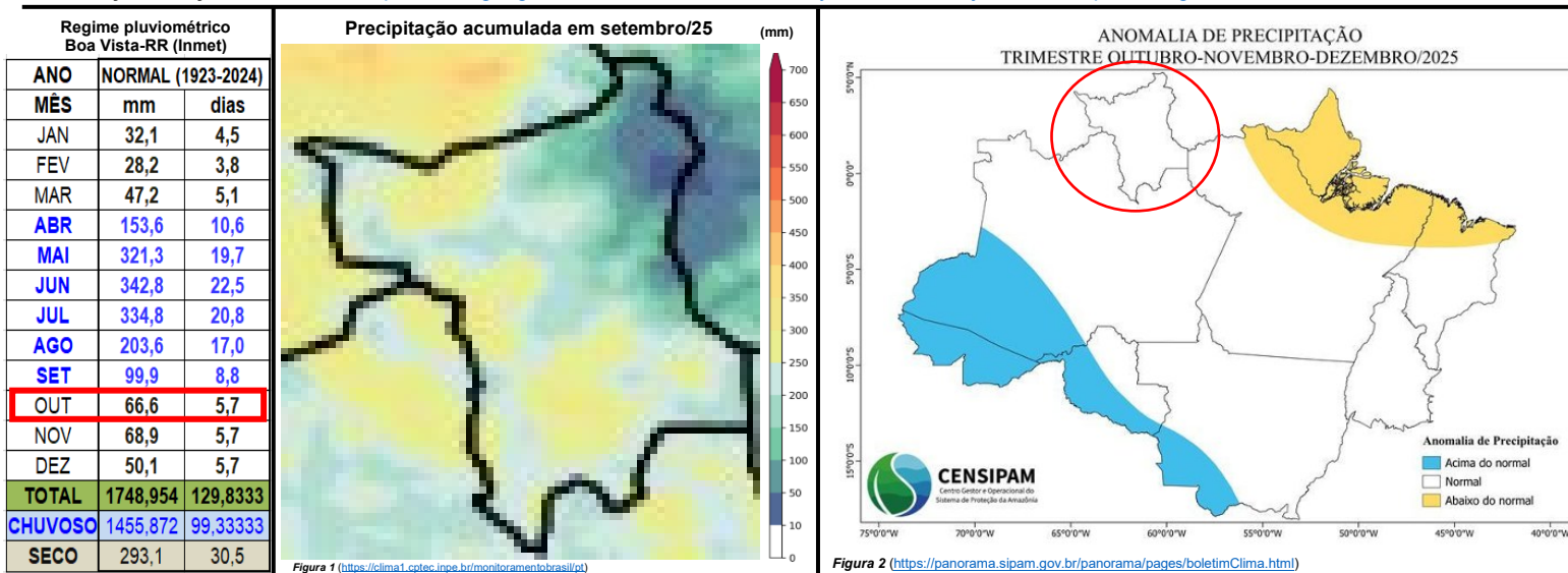
Figura 1 ( https://clima1.cptec.inpe.br/monitoramentobrasil/pt )
