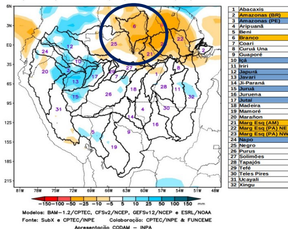
PREVISÃO SUBSAZONAL—MULTIMODELO CALIBRADO Anomalia (mm) de Precipitação Acumulada (14 Dias) Período: 23/07/2025 – 05/08/2025
