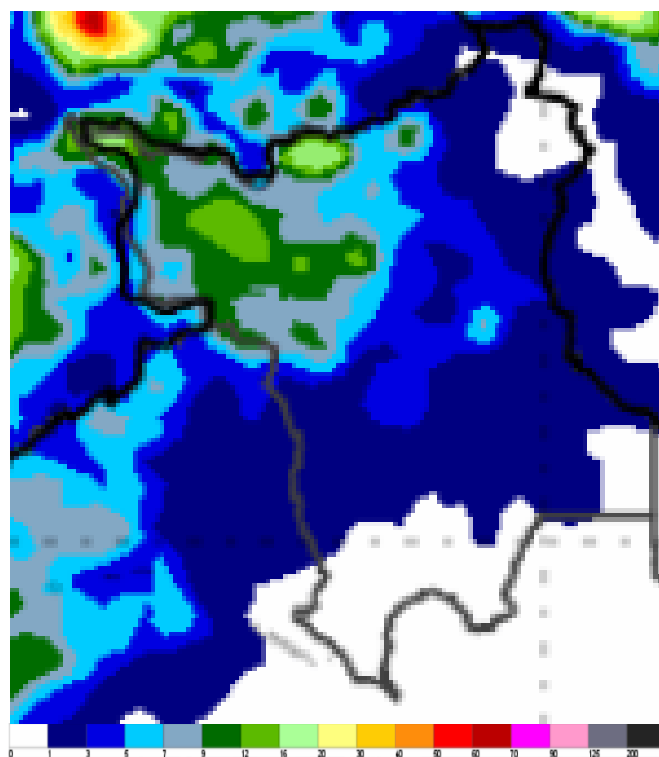
Figure 3 – Modelo de precipitação COSMO (7 x 7km): https://vime.inmet.gov.br/CO
