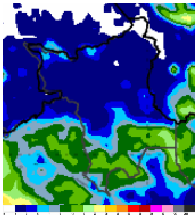
Figura 3 – Modelo de precipitação COSMO (7 x 7km):
